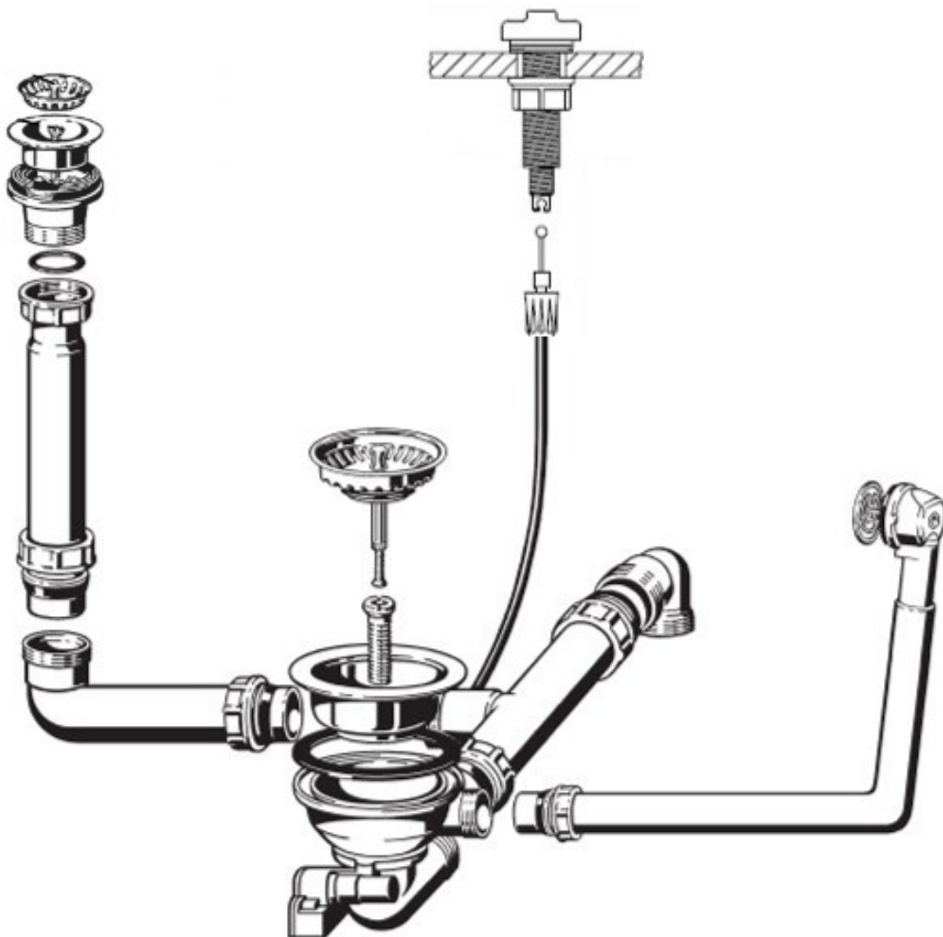
Ablaufgarnitur mit Excenterbetätigung 1 x 3 1/2"
