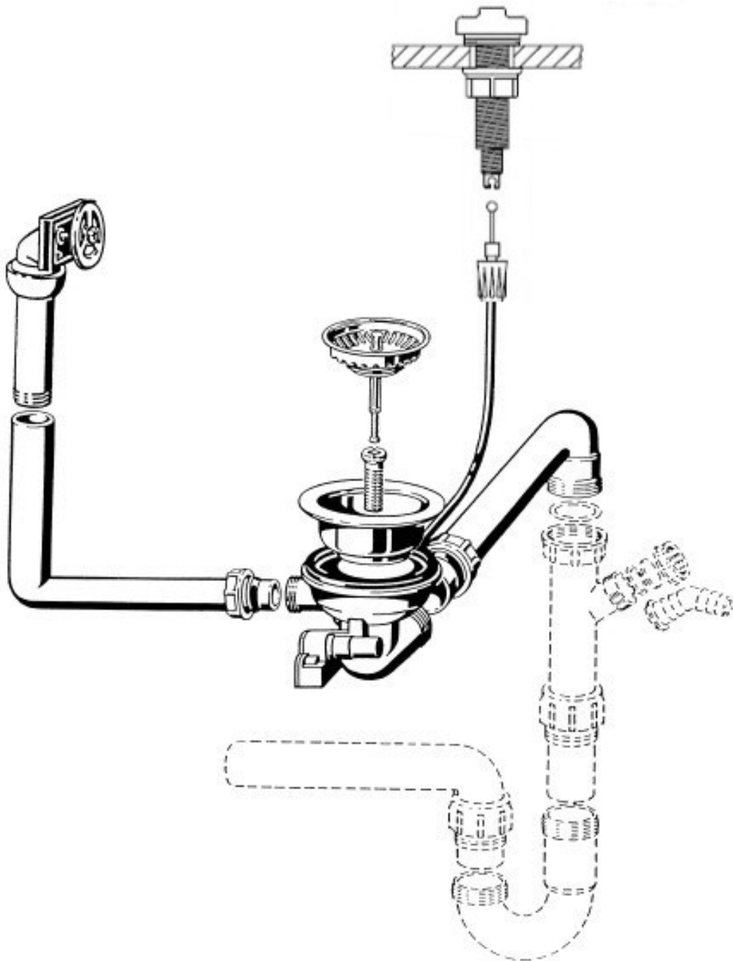
Ablaufgarnitur mit Excenterbetätigung 1 x 3 1/2"
