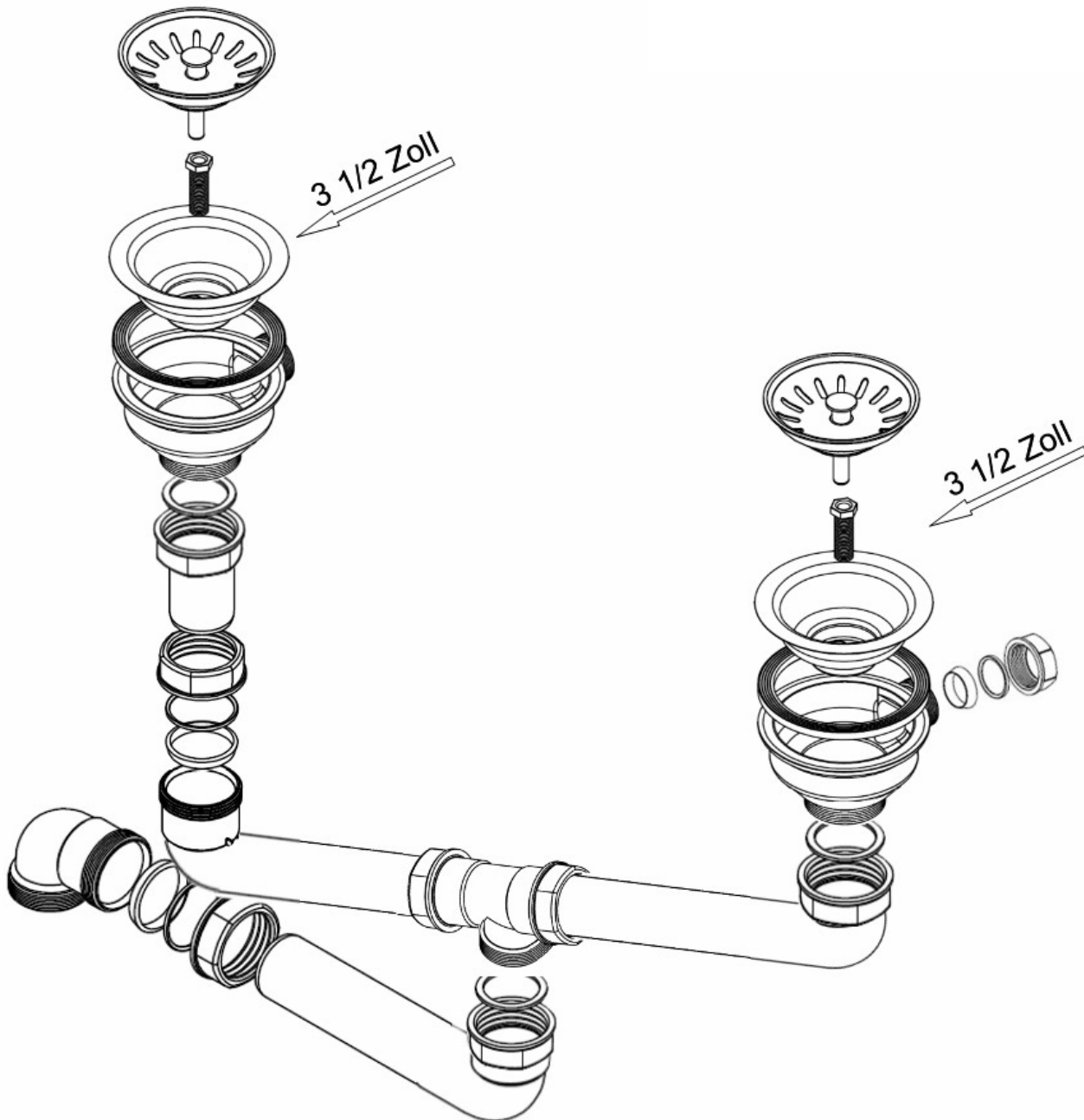
Ablaufgarnitur mit Handbetätigung 2 x 3 1/2"
